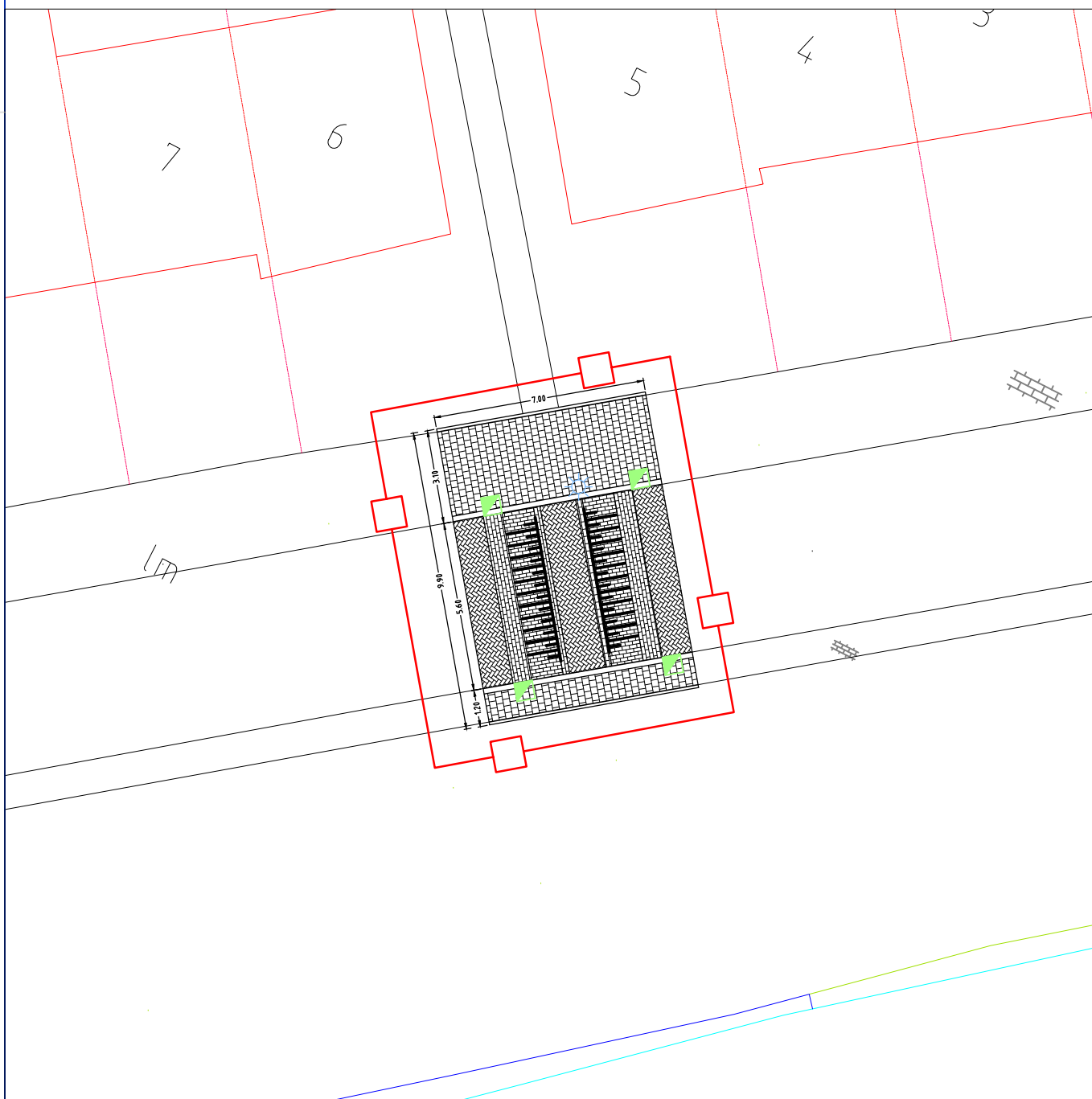
Tekening 11 : Drempel Jan van Galenstraat, 6/5 Schaal 1:200
