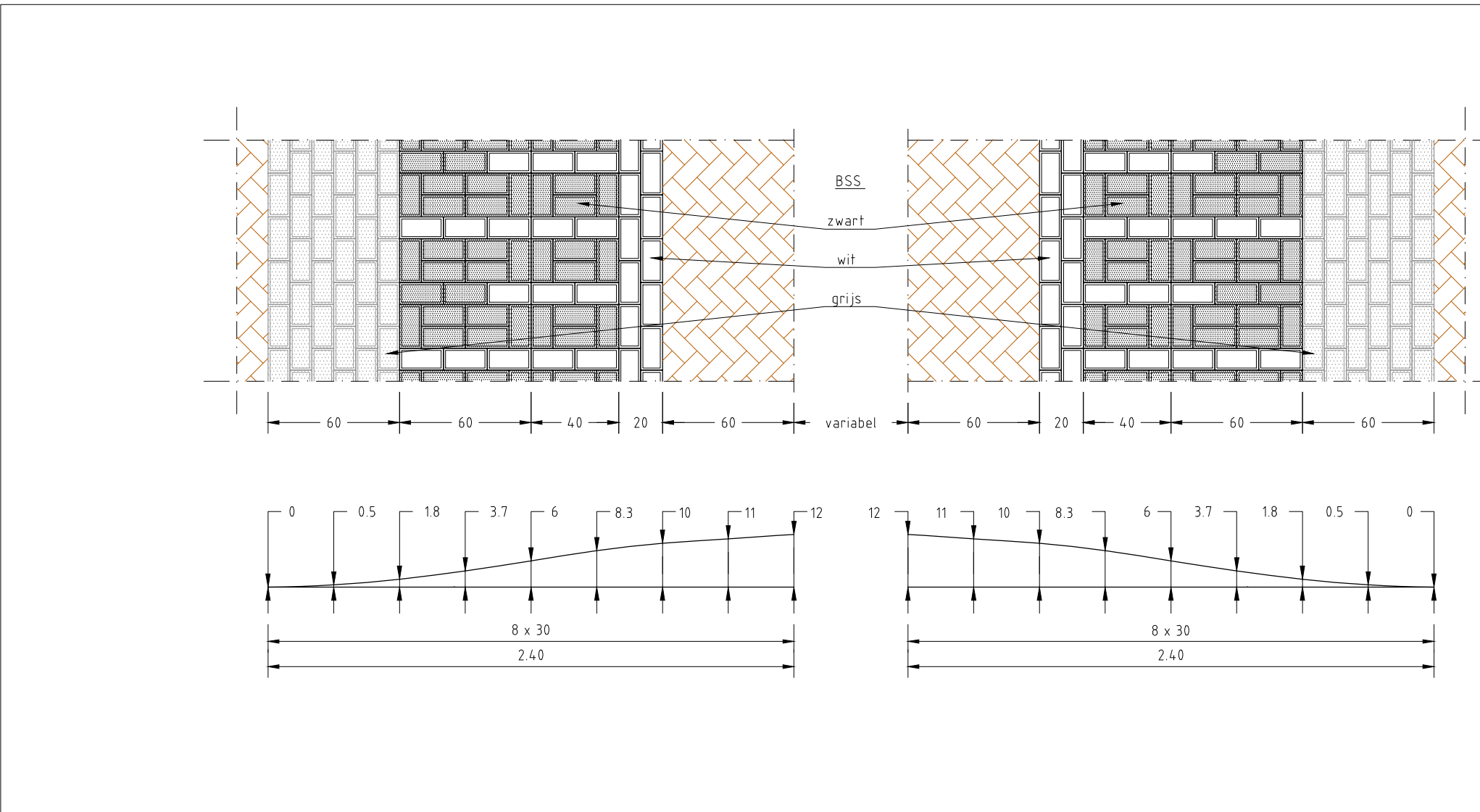
Detailtekening drempel schaal 1:25
