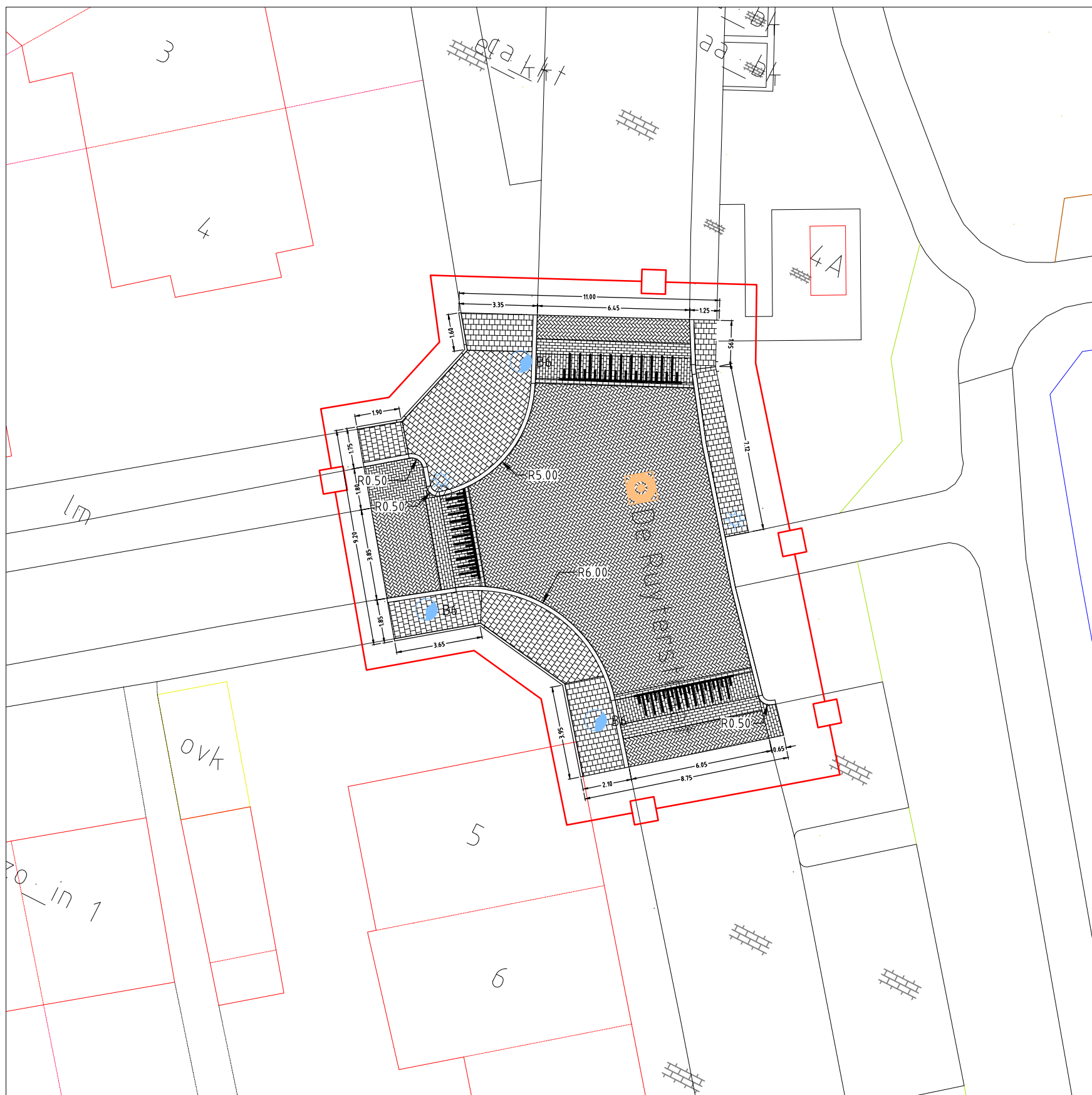
Tekening 5 : Plateau Trompstraat, De Ruyterstraat Schaal 1:200
