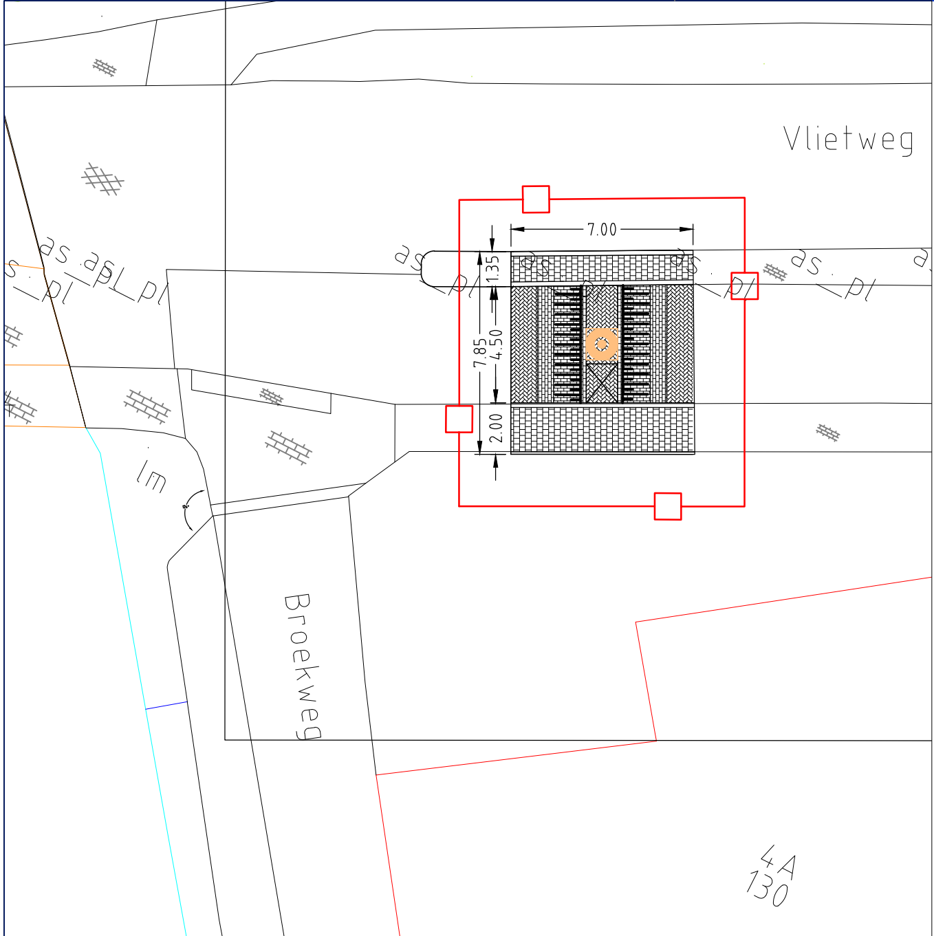
Tekening 1 : Drempel Vlietweg, 130 Schaal 1:200
