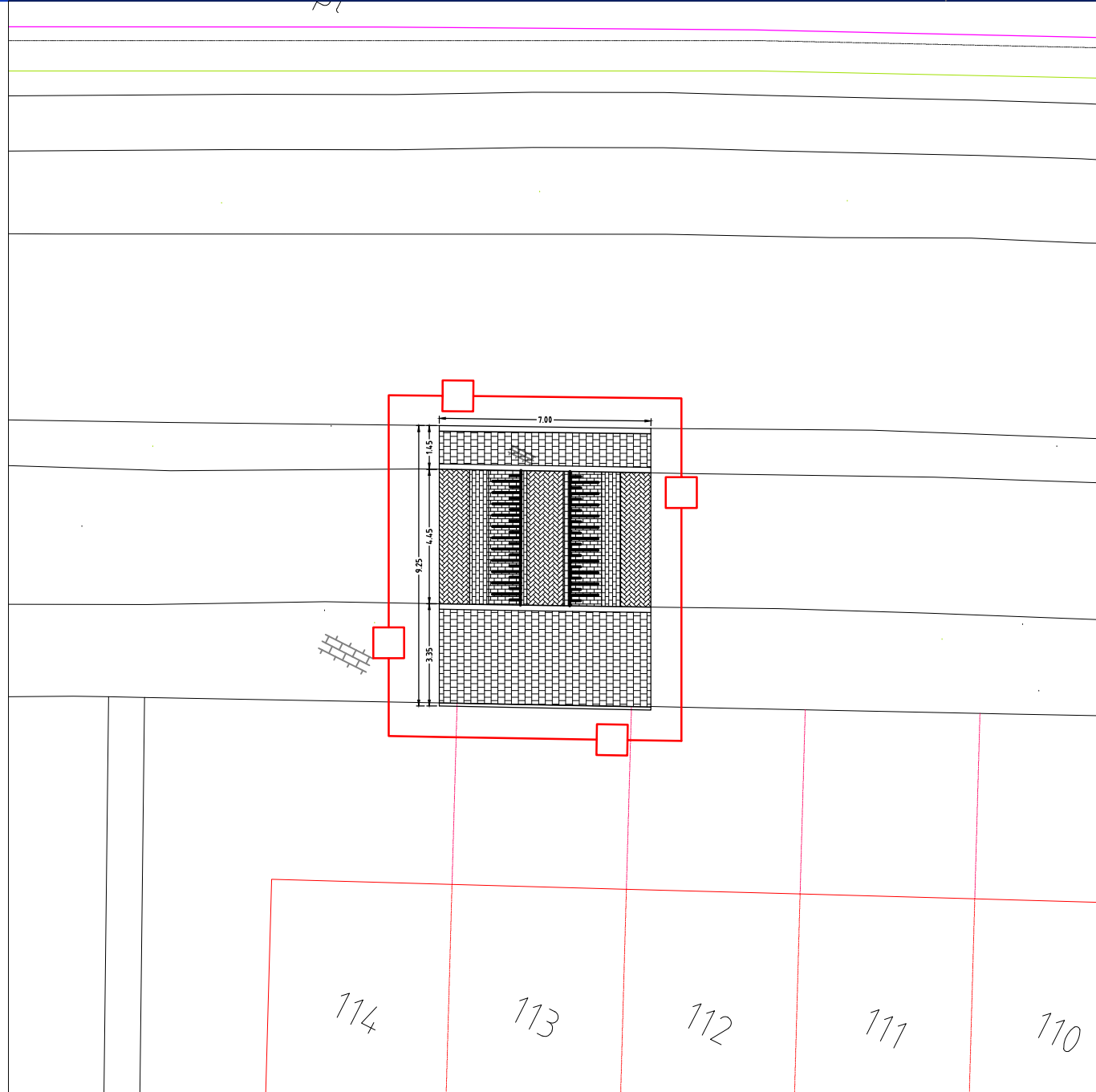
Tekening 3 : Drempel Vlietweg, 113 Schaal 1:200
