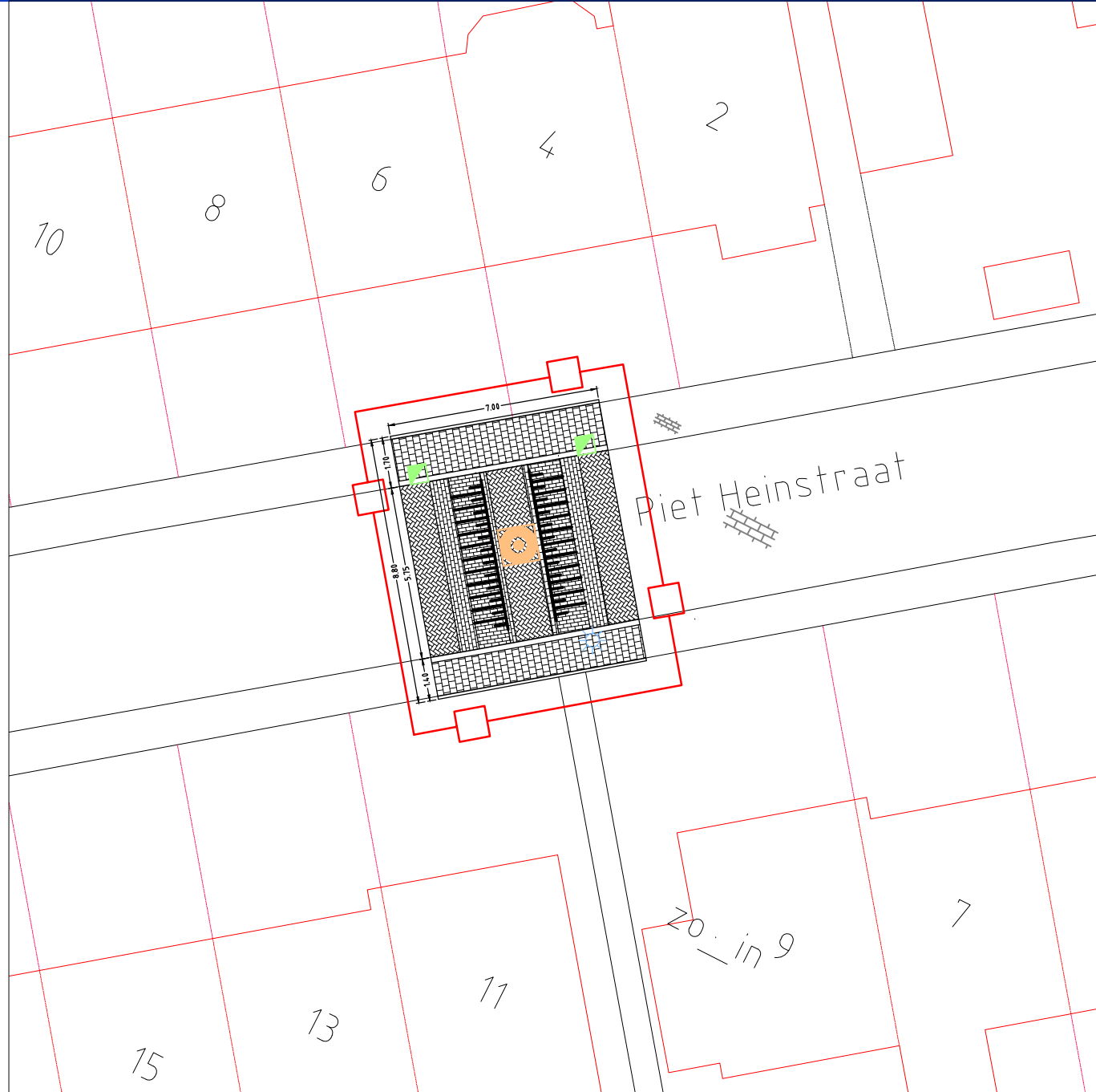
Tekening 9 : Drempel Piet Heinstraat, 11/9 Schaal 1:200
